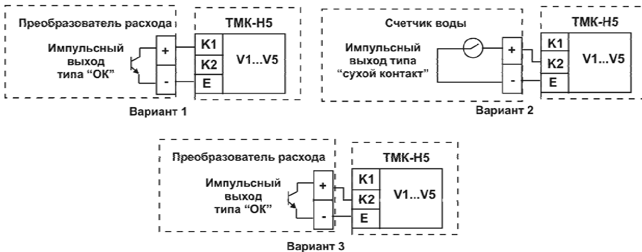
Рисунок Г.3 - Схема подключения преобразователей расхода и счетчиков воды к TMK-H5
