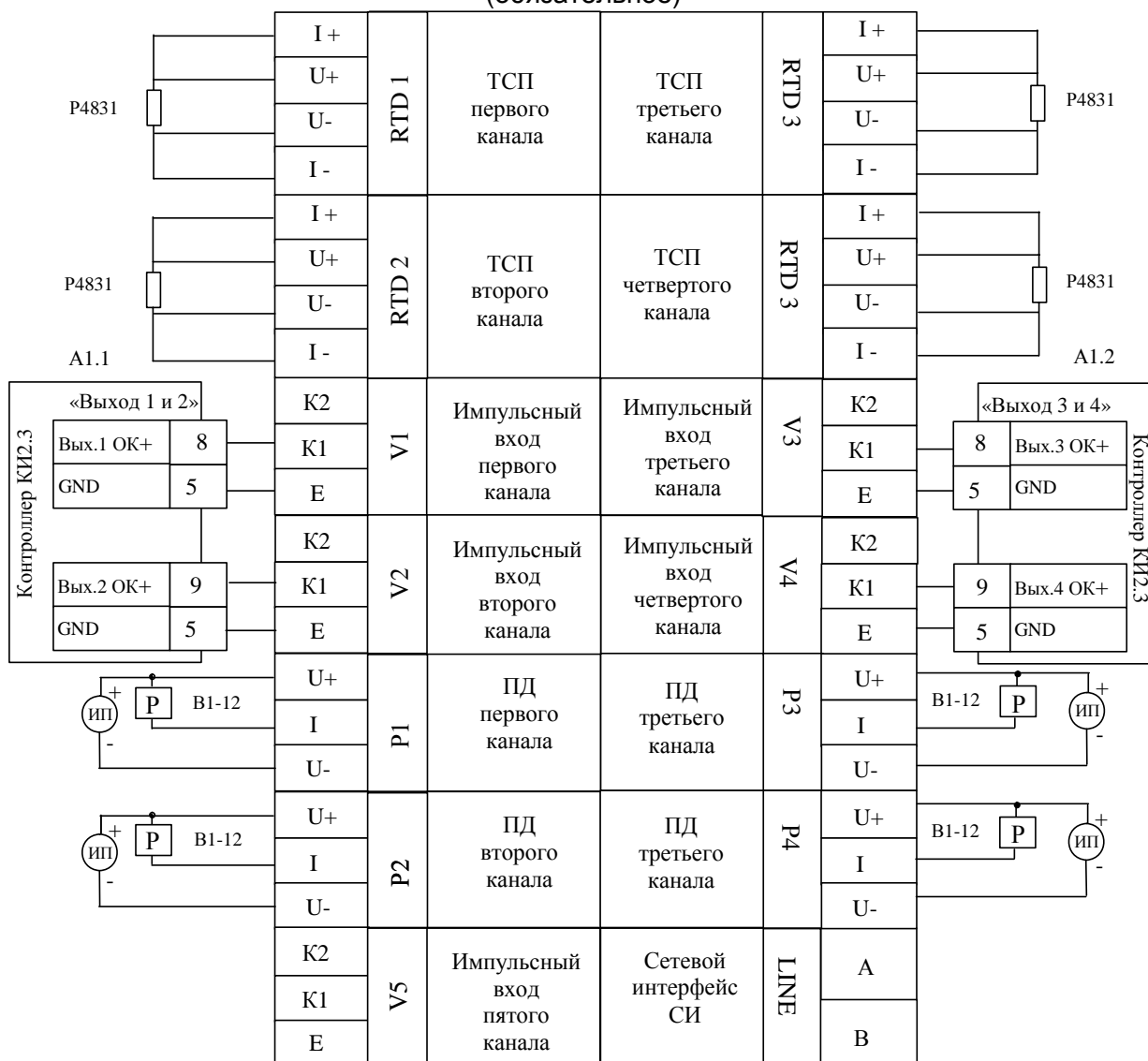
Рисунок Е.1 - Схема подключения вычислителя ТМК-5 к приборам и оборудованию при его поверке (P - калибраторы тока, ТСП- термометр сопротивлений, ПД – преобразователь давления, ИП – источник питания стабилизированным напряжением U_{н}=24В I_{макс}= 50мА )
