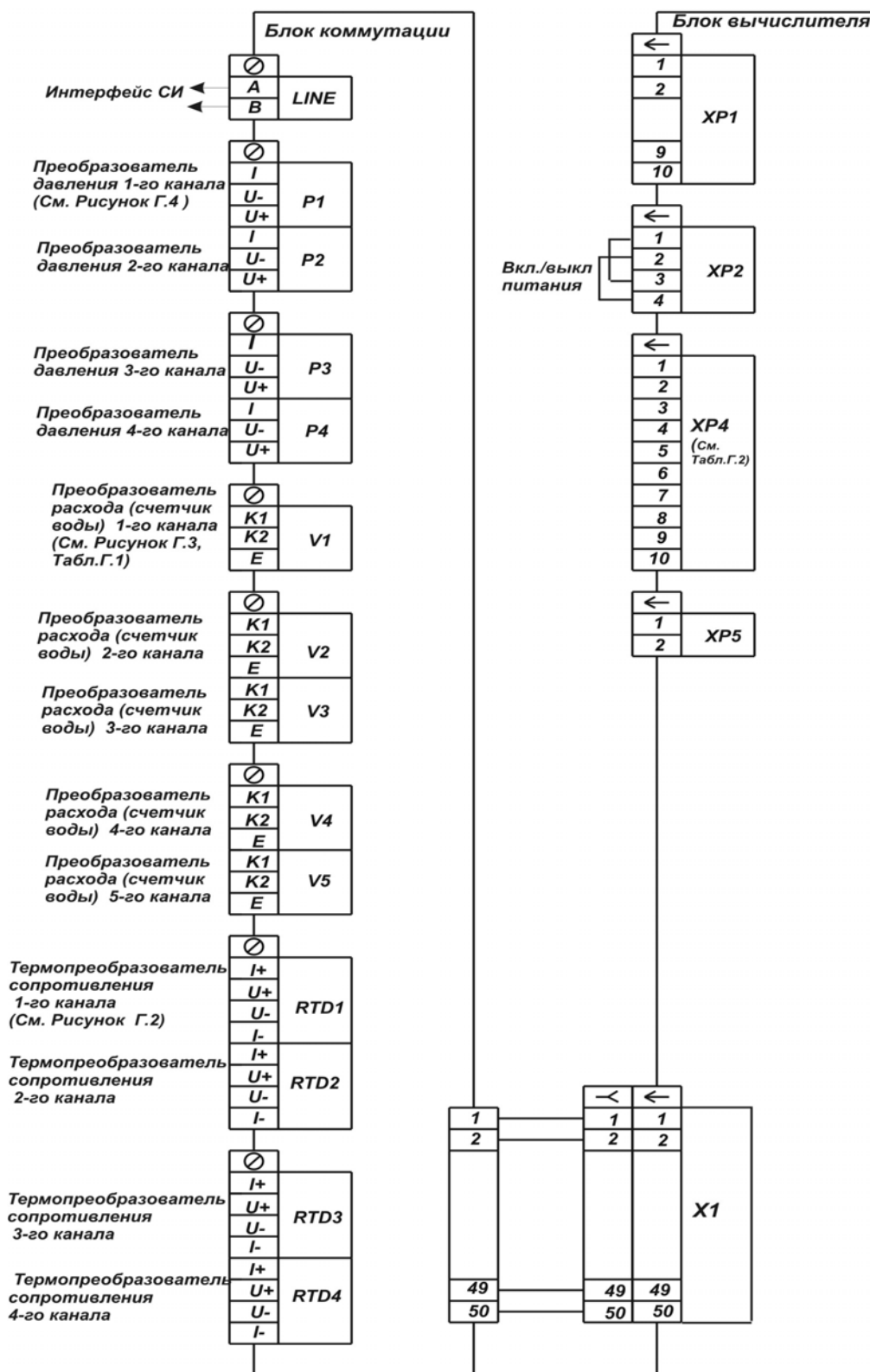
Рисунок Г.1 – Схема подключения внешних устройств к ТМК-Н5
