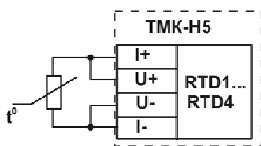
Рисунок Г.2 - Схема подключения термопреобразователей к TMK-H5
